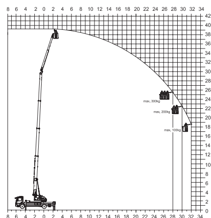
Praca z podestem (HA 3/300) przy 1-krotnie wysuniętym wierzchołku
